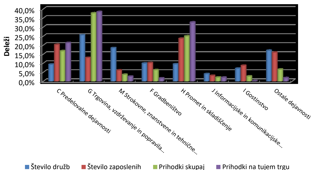
Graf 3: Struktura pomembnejših podatkov o poslovanju v letu 2020 po pomembnejših dejavnostih
