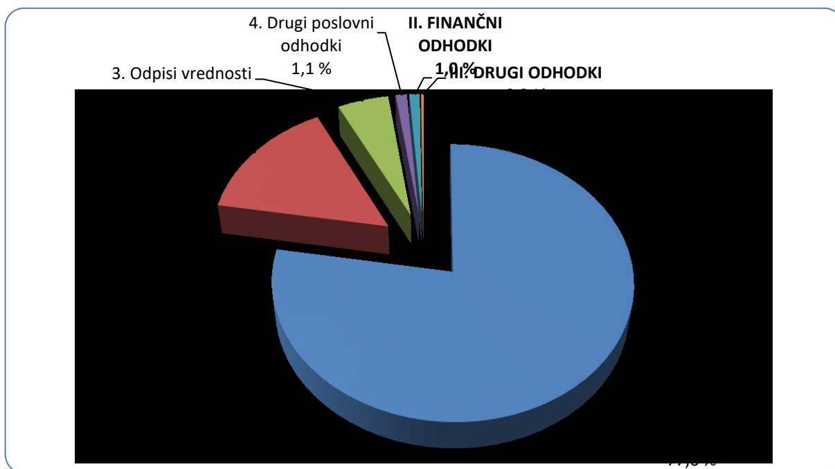
Graf 2: Struktura posameznih vrst odhodkov
