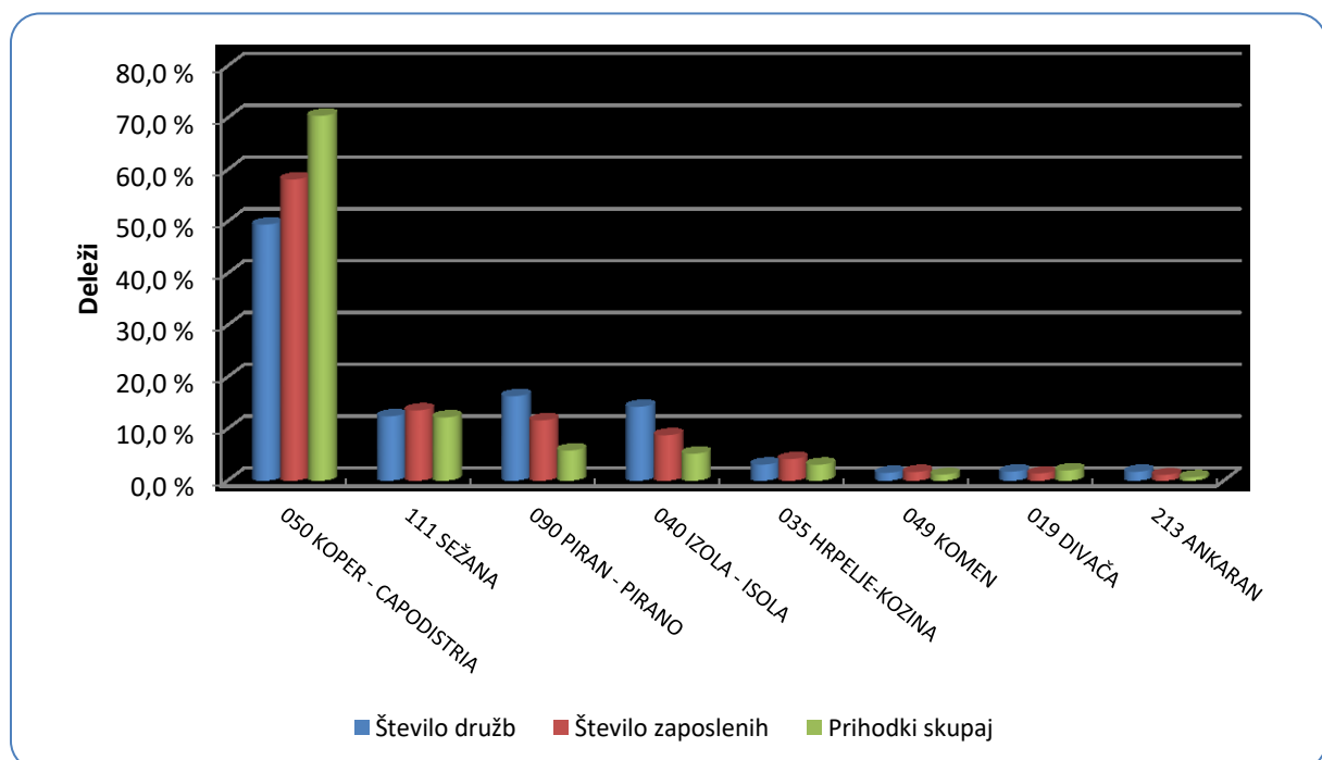
Graf 4: Struktura pomembnejših podatkov o poslovanju družb v letu 2020 po občinah
