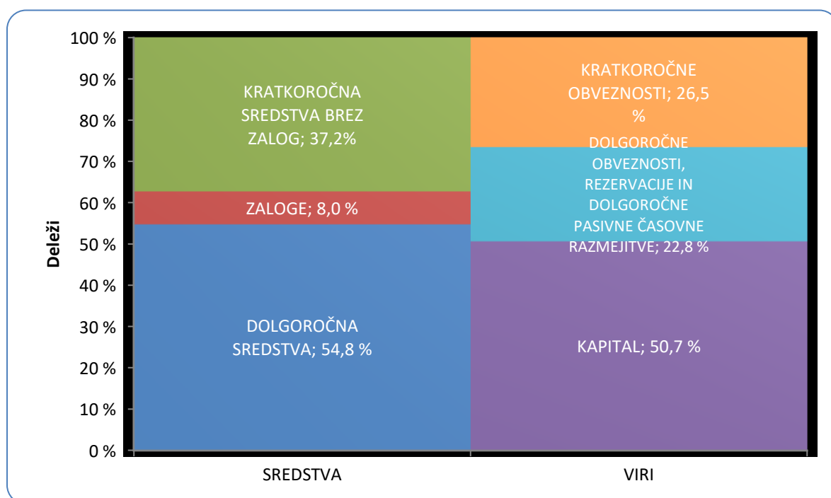
Graf 6: Struktura sredstev in obveznosti do virov sredstev družb na dan 31. 12. 2020
