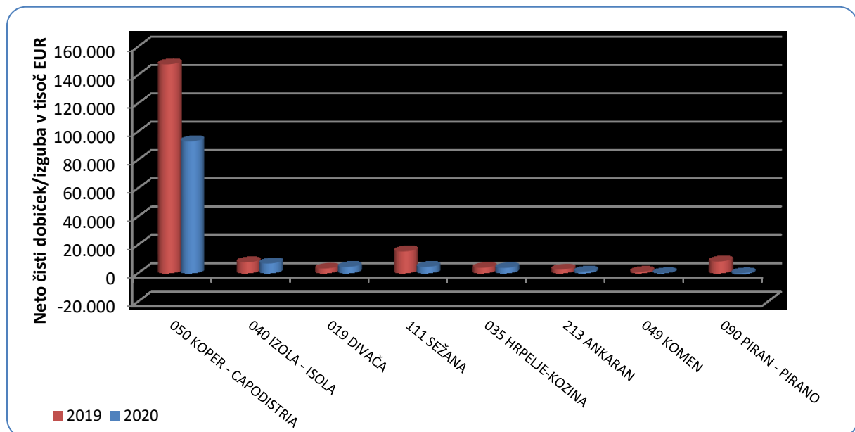
Graf 5: Prikaz neto čistega dobička/izgube družb v letu 2019 in 2020 po občinah
