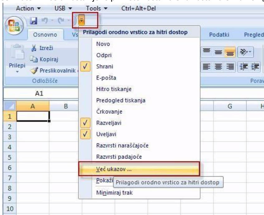
Slika 4 Pot do nastavitve za nastavitve makrov
